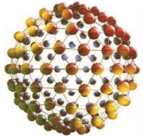
Cadena lineal de la molécula
